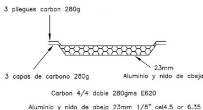
Dibujo N°255-14
